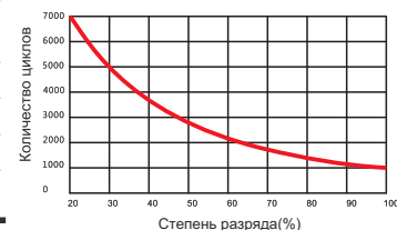
Зависимость циклов от глубины разряда
